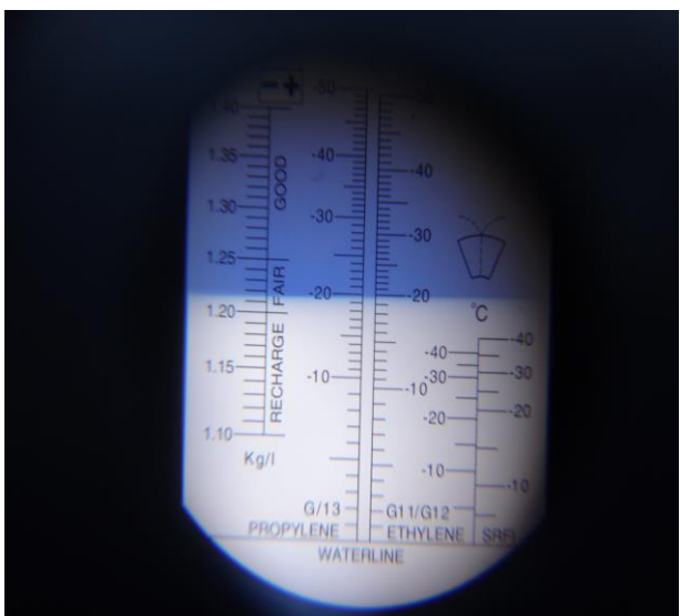
バッテリー比重写真 (1.22)
