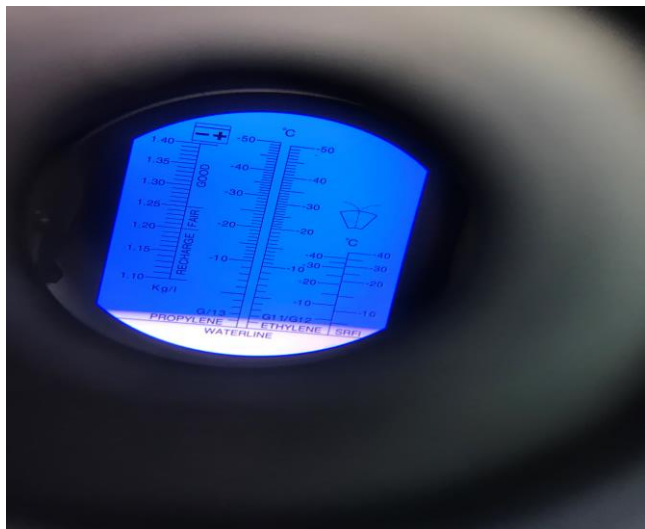
ウォシャータンク濃度状況写真
