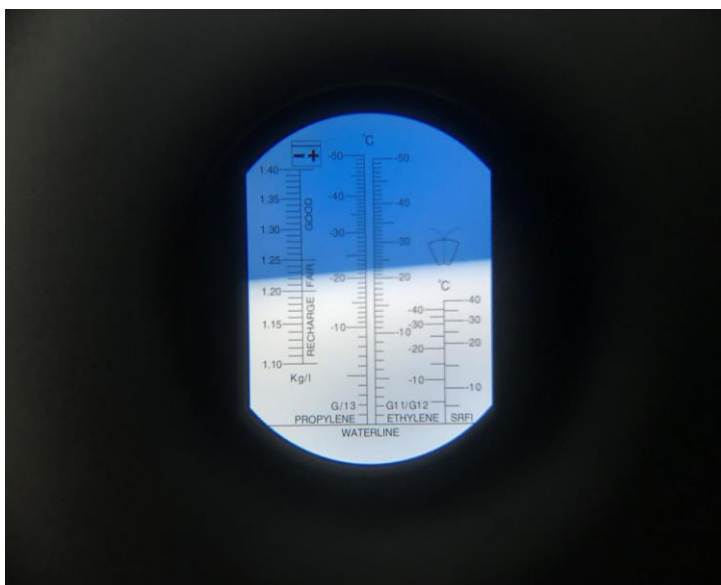
バッテリー比重 (1.22)
