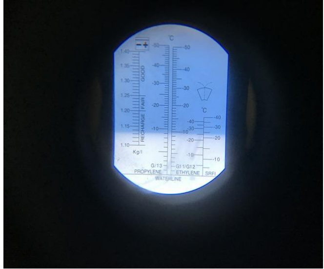
LLC濃度 (-10℃)
