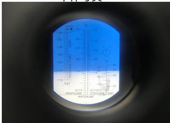
バッテリー比重 (1.15)
