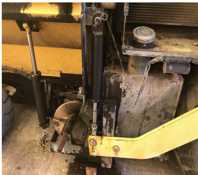
スクリーンベース昇降シリンダーOH
