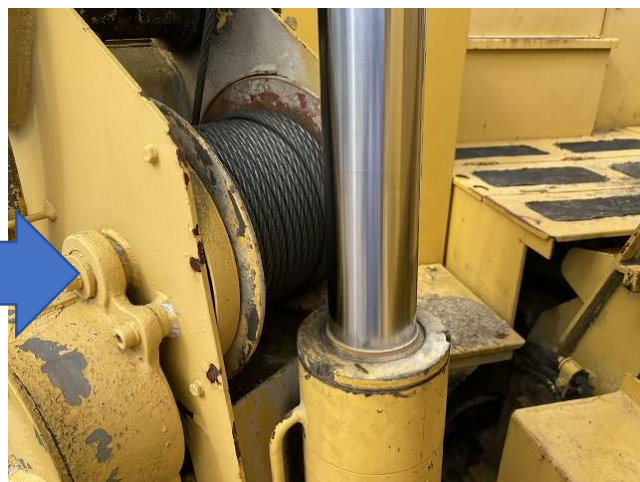
クレーン起伏シリンダシール交換
