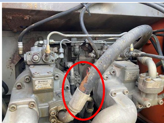
メインポンプ戻りホース劣化
