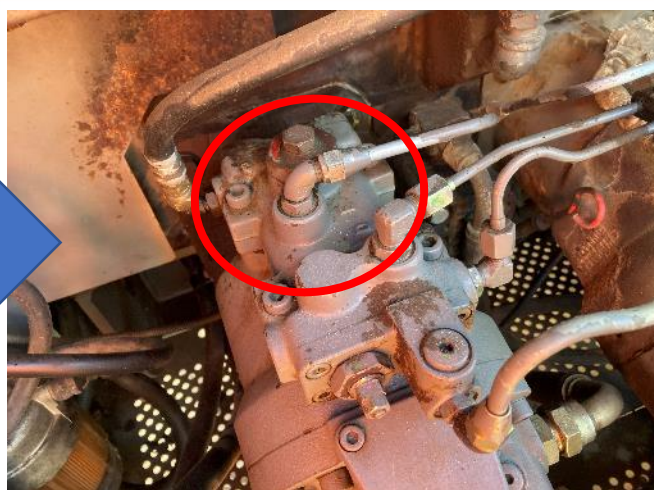
油圧ポンプレギュレーター油漏れ修理
