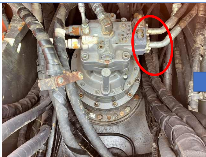
旋回モーターバルブ面油漏れの為修理
