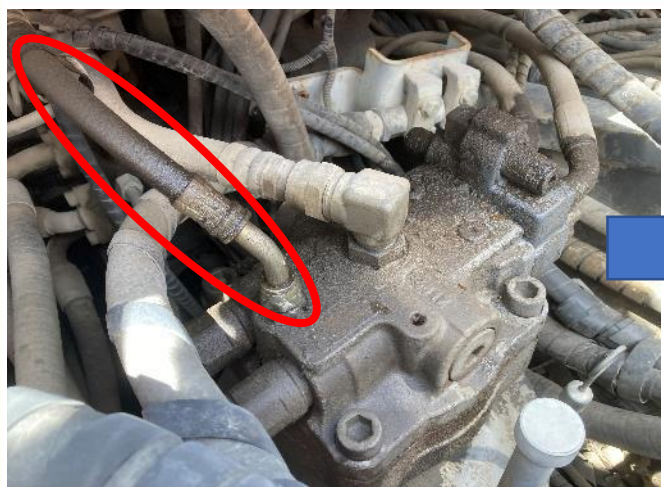
コントロールバルブ 油圧ホース交換
