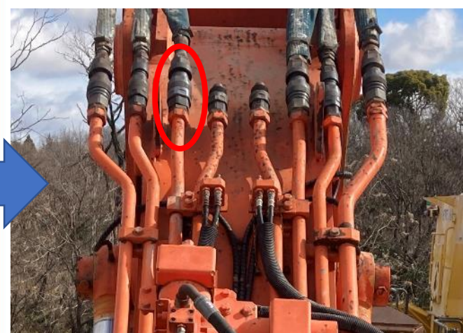
フロントホースカプラ交換
