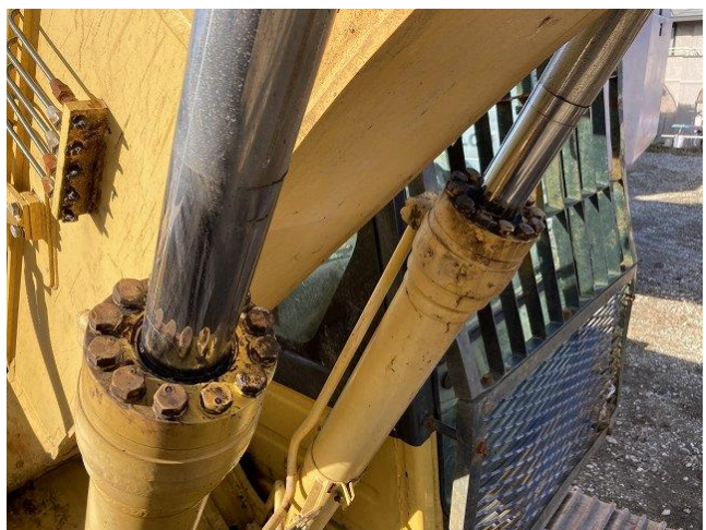
ブームシリンダー油漏れ(両側)
