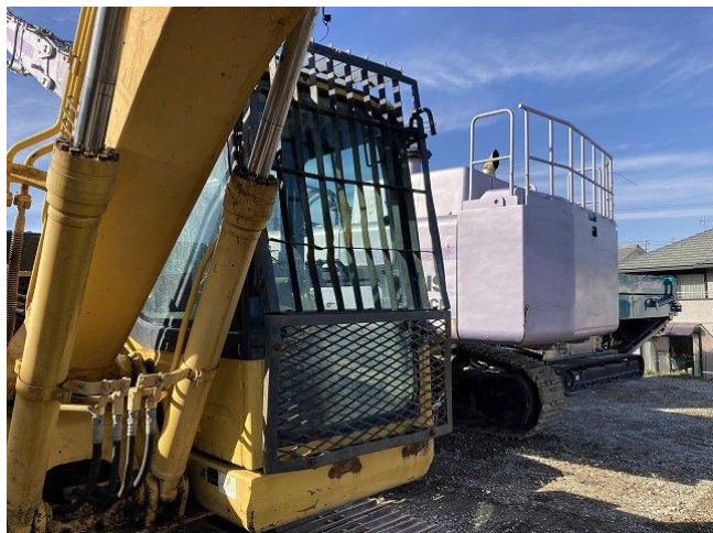
フロントガード変形
