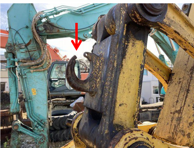
フックラッチ欠損
