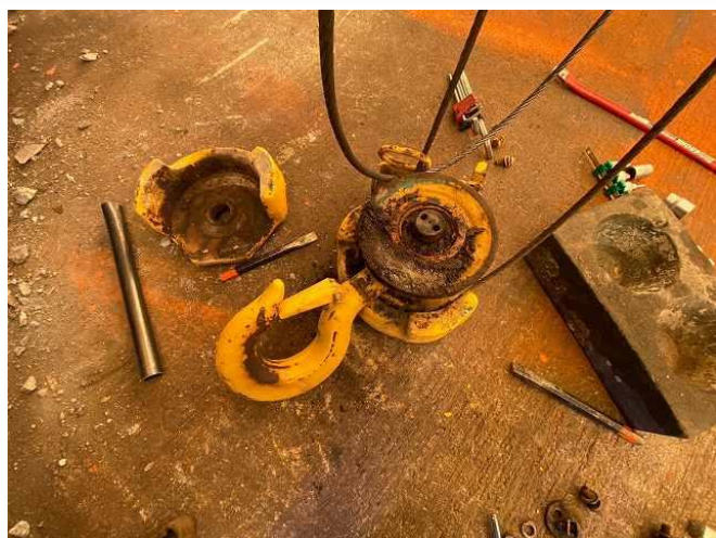
クレーンフックシーブ不動の為交換
