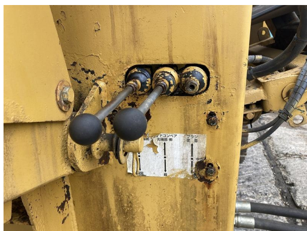
サイドCV操作レバーより油漏れ
