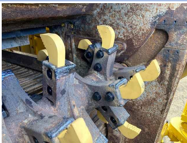
ソイルカッター全数新品交換
