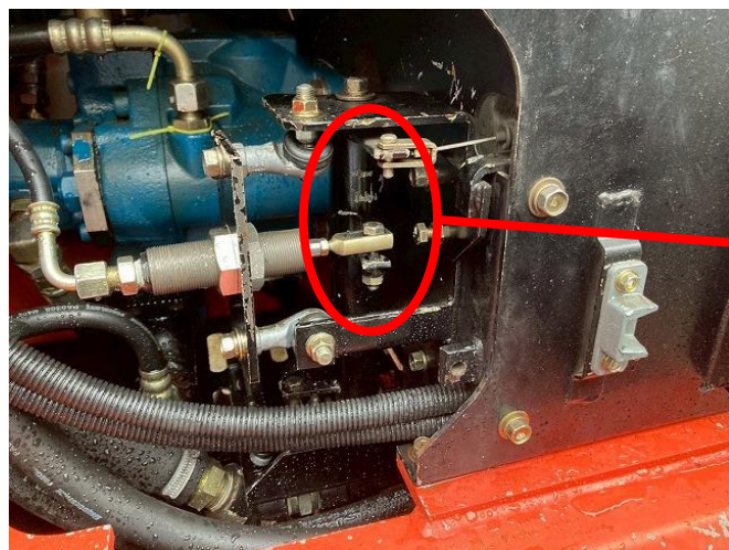
アクセルワイヤー取付リンケージ固着修正
