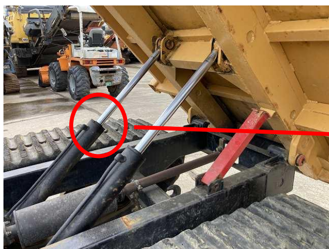
ダンプシリンダー油漏れ②(右側)
