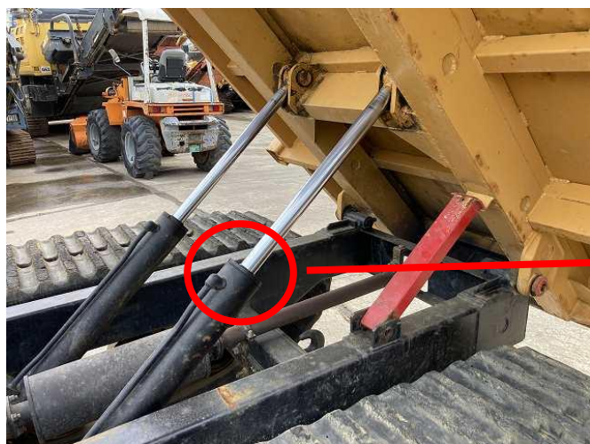
ダンプシリンダー油漏れ①(左側)
