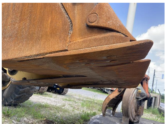
バケットツース摩耗(反転済)
