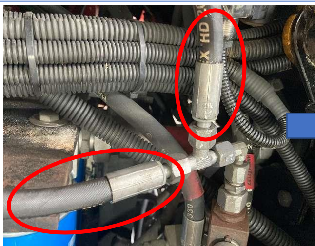
バルブ間油圧ホース2本交換(2024年10月作業)
