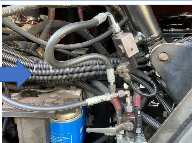
バルブ間油圧ホース2本交換(2024年10月作業)
