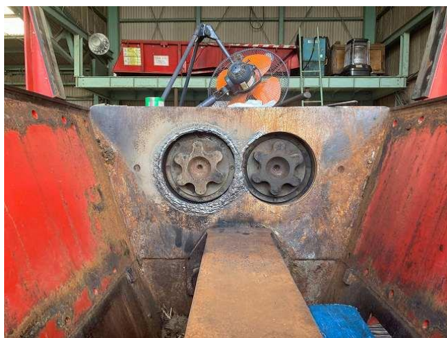
クローバーカップリング溶接肉盛り(2024年10月作業)
