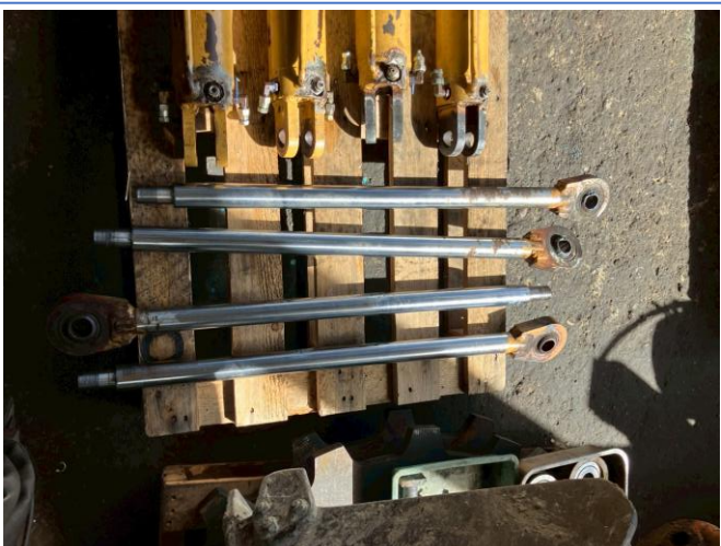
コンベア調整シリンダOH(4本),ロッド再生
