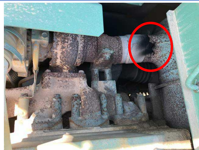
マフラーパイプ継ぎ目付近破れ
