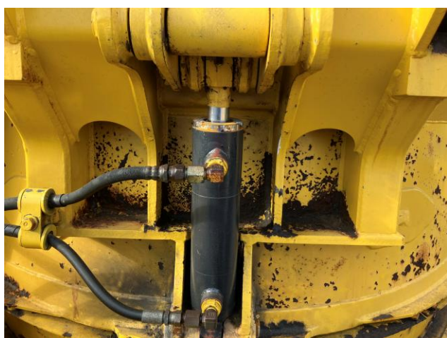
タブカバー開閉シリンダー オイル漏れ修理
