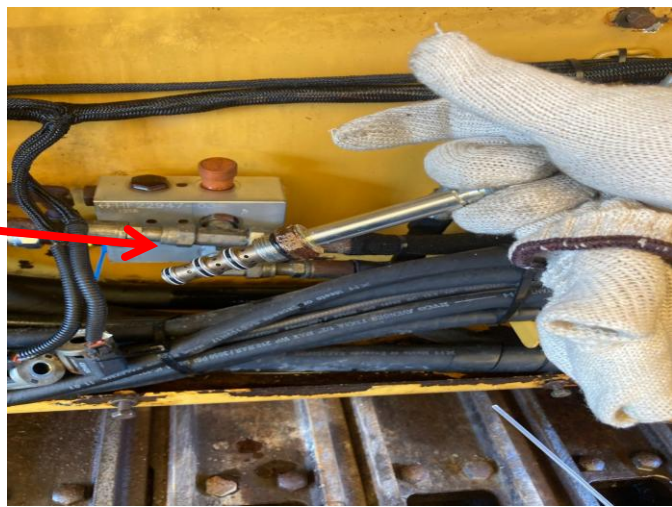
飛散防止カバー不動の為ソレノイド交換
