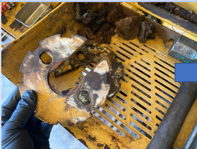
ハンマーミル回転測定プレートがたつきの為交換、回転センサー交換
