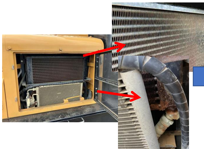
オイルクーラー交換
