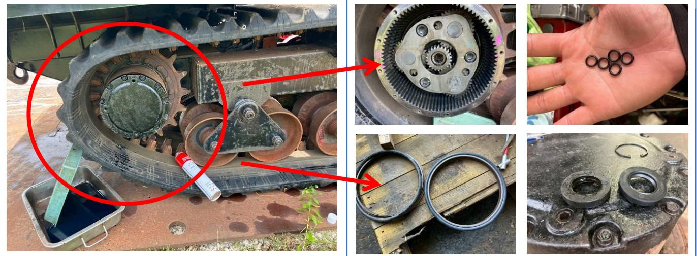
走行モーター及び減速機分解シール類交換(左側)
