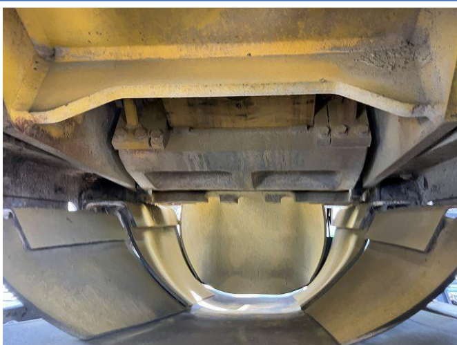
トグルプレート交換
